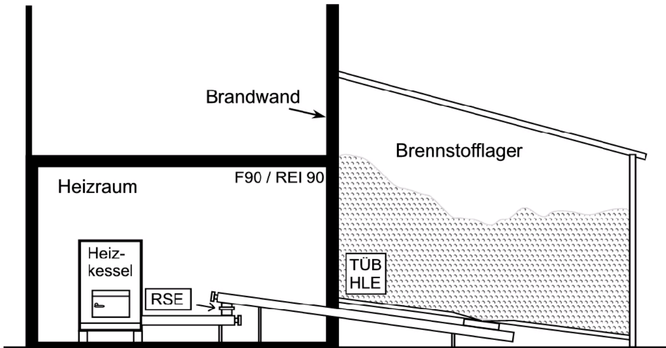
Bild 4: Automatische Austragung aus dem angebauten Brennstofflager (5.1.2), Heizleistung \leq 400 \text{ kW} und Lagermenge > 50 \text{ m}^3 \leq 200 \text{ m}^3 , Brennstoff gemäß Punkte 3.1 (Hackgut)
