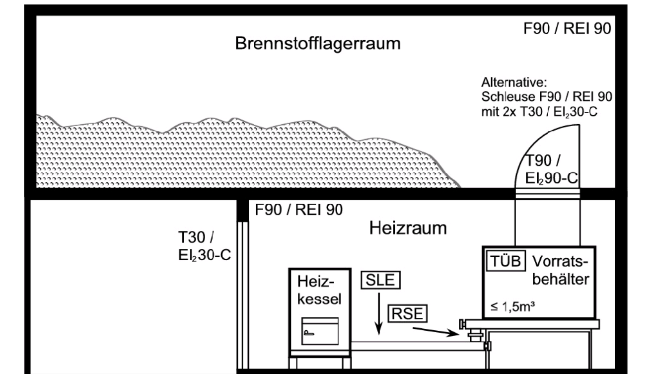
Bild 15: Vorratsbehälter \leq 1,5\text{ m}^3 im Heizraum (5.1.3) mit Verbindung zum darüber liegenden Brennstofflager (5.1.3), Heizleistung \leq 150\text{ kW} , Brennstoff gemäß Punkt 3.3 (sonstige Holzreste)
