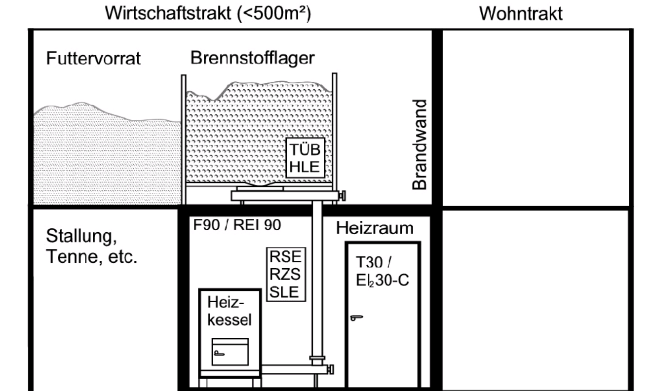
Bild 5: Automatische Austragung aus dem Brennstofflager (5.1.2) im Wirtschaftstrakt (Bergeraum), Heizleistung \leq 150 \text{ kW} und Lagermenge \leq 200 \text{ m}^3 , Brennstoff gemäß Punkte 3.1 (Hackgut)
