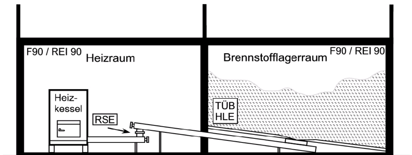
Bild 3: Automatische Austragung aus dem Brennstofflagerraum (5.1.3), Heizleistung \leq 400 \text{ kW} , Lagermenge > 50 \text{ m}^3 \leq 200 \text{ m}^3 - Brennstoff gemäß Punkt 3.1 (Hackgut)
