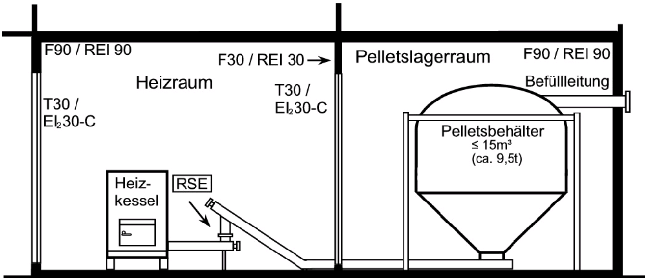
Bild 9a: Automatische Austragung aus dem Brennstofflagerraum (5.1.3, brennbarer Behälter im Lagerraum), Heizleistung \leq 150 kW und Lagermenge \leq 15 m 3 (ca. 9,5 to), Brennstoff gemäß Punkt 3.2 (Pellets)
