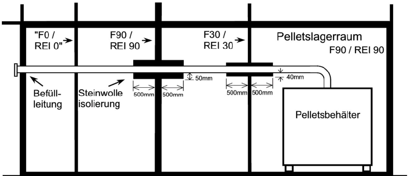
Bild 17: Ausführungsbeispiel einer Befüllleitung (Stahlrohr < DN 150 ) welche durch brandabschnittsbildende Bauteile geführt wird. Detailsausbildung im Bereich von Wanddurchdringungen bei Verwendung von Steinwolleisierungen: Steinwolle: nichtbrennbar, Raumgewicht ca. 150 kg/m 3 , Schmelzpunkt > 1000^\circ C F 30 (REI 30): - Mindestlänge der Isolierung an beiden Seiten: l = 500 mm - Mindestdicke der Isolierung: d = 40 mm F 90 (REI 90): - Mindestlänge der Isolierung an beiden Seiten: l = 500 mm - Mindestdicke der Isolierung: d = 50 mm Die Isolierungen sind durch die Öffnungen zu führen, der verbleibende Restspalt zu vermörteln. Die Isolierungen sind an beiden Seiten der Wand mit Bindedraht zu sichern. Die Befüllleitungen sind in geeigneter Weise zu fixieren (Deckenabhängungen mind. M 10).
